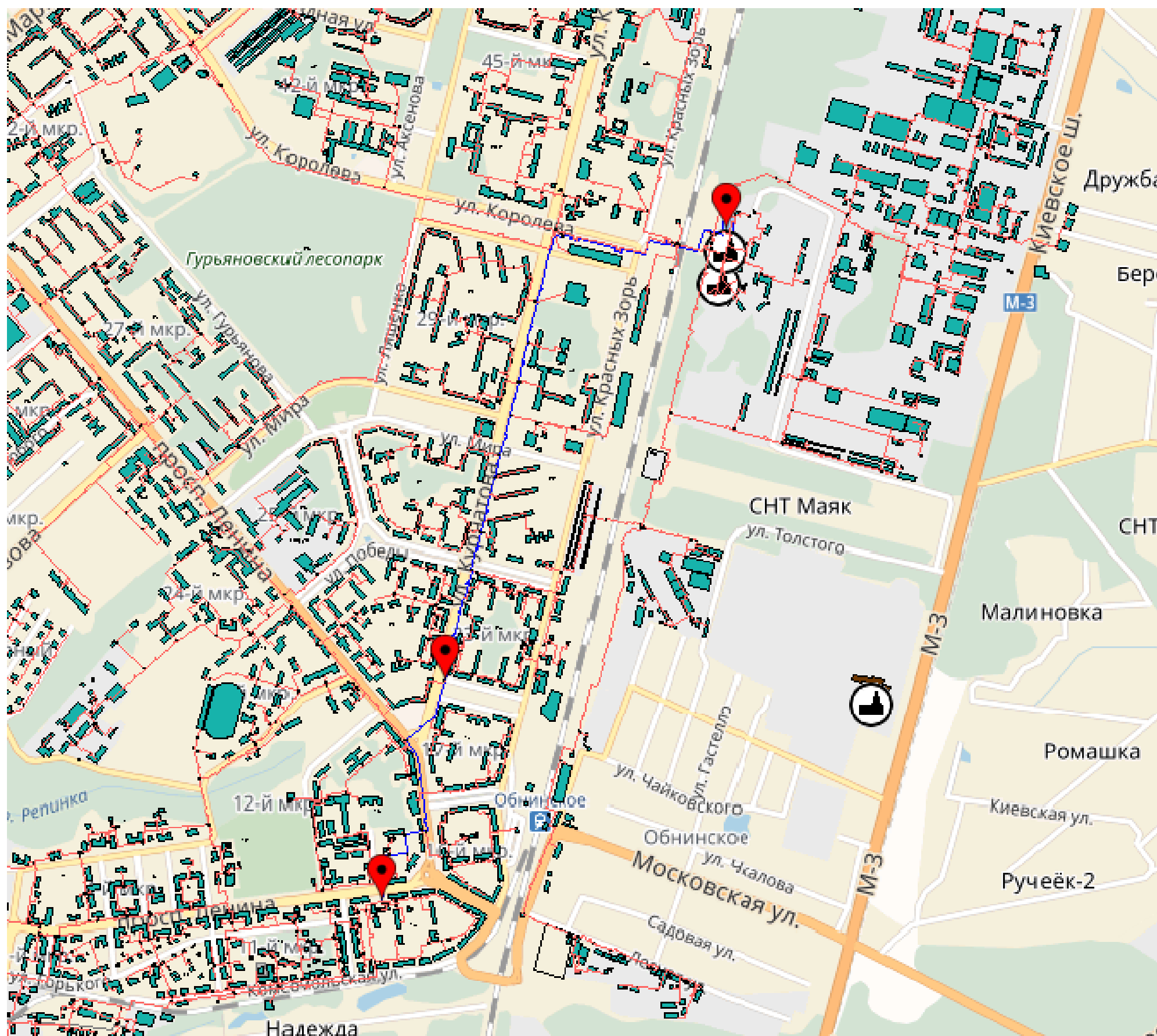
Рисунок 3 - Путь для построения пьезометрического графика магистрального вывода от котельной МП «Теплоснабжение» (2 очередь) до ТК-6
